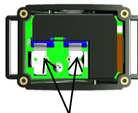
Reset : relier les 2 supports de pile Fig. 7
